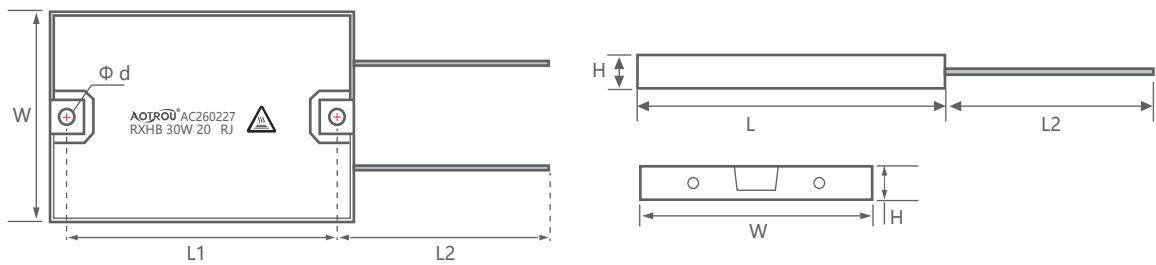
RXHB 产品尺寸图 (RXHB Product Size)
